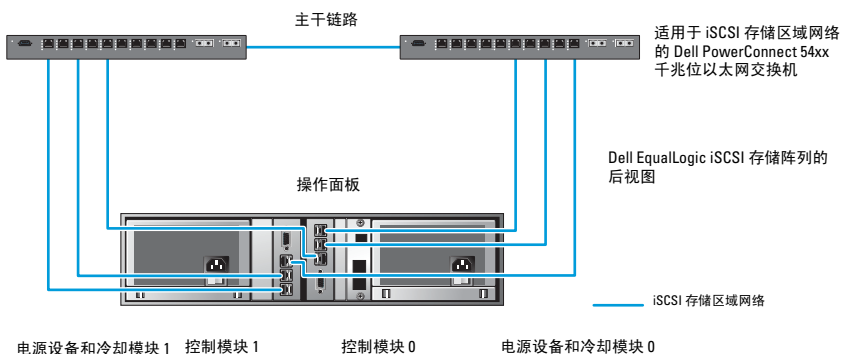
图 5-1. 推荐的网络配置
